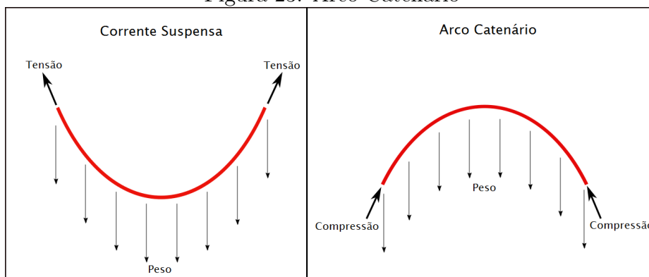
Figura 23: Arco Catenário
