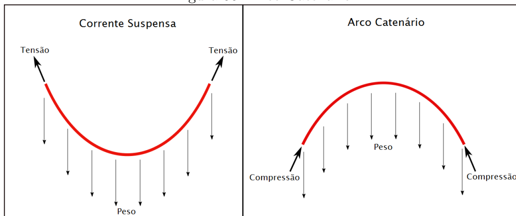
Figura 56: Arco Catenário
