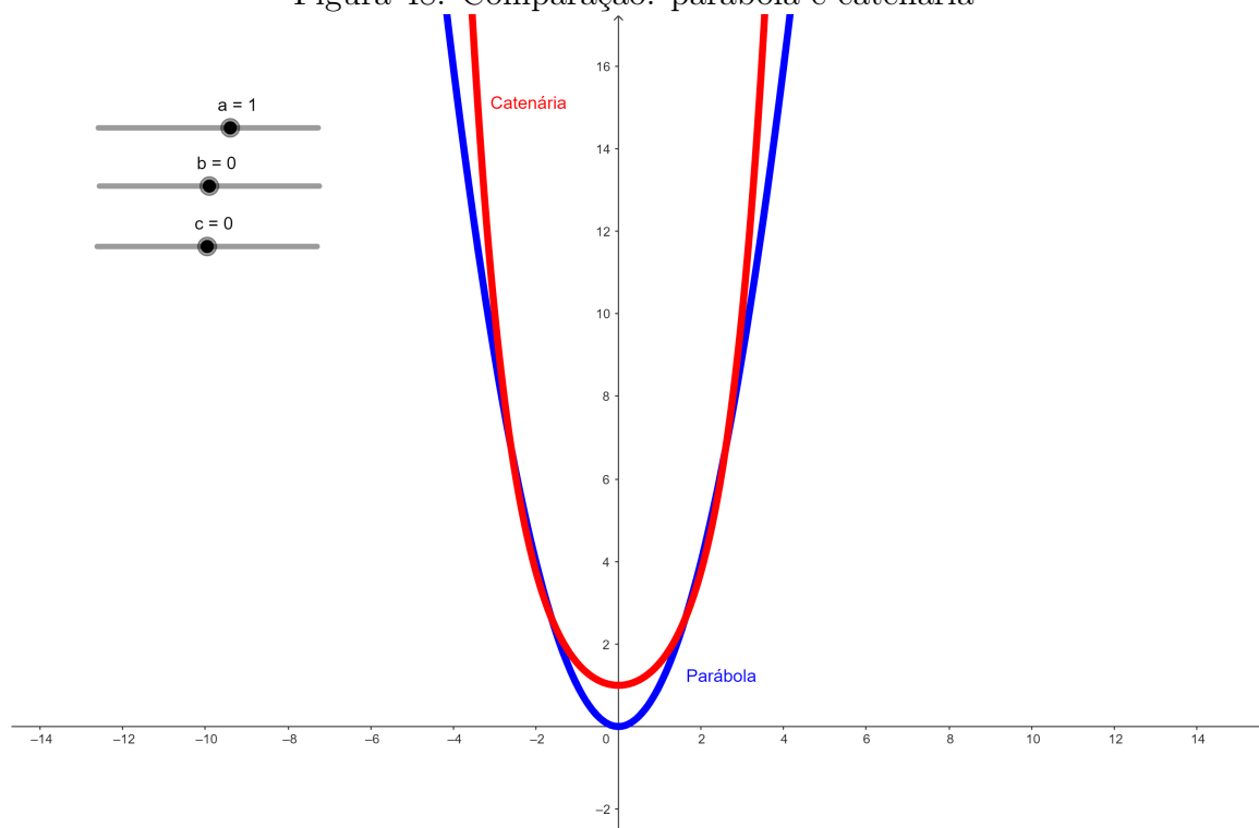
Figura 48: Comparação: parábola e catenária
