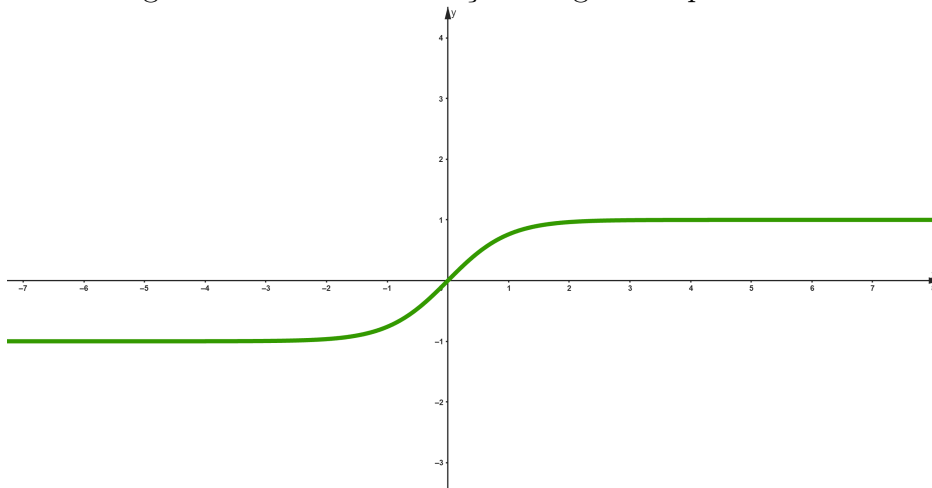
Figura 16: Gráfico da função Tangente Hiperbólica.
