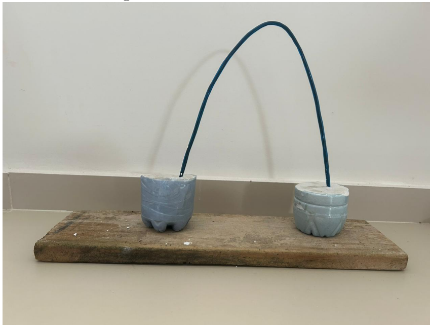
Figura 80: Parábola construída
