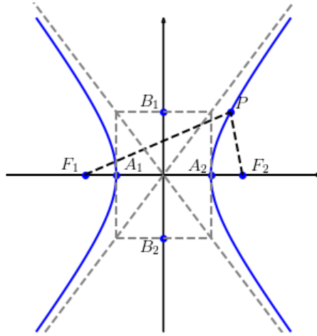
Figura 4: Assíntotas da hipérbole
