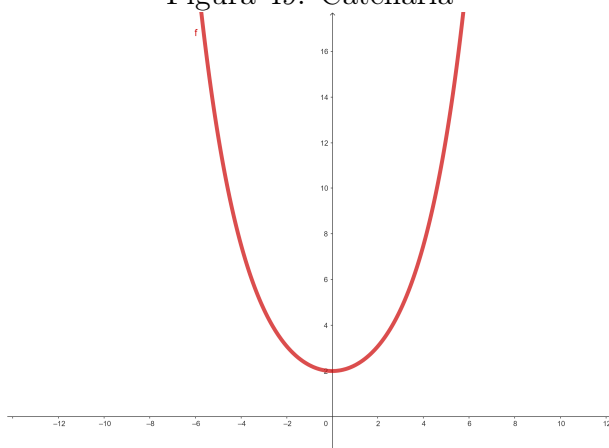
Figura 49: Catenária
