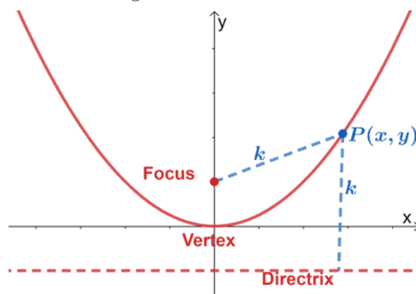
Figura 40: Parábola
