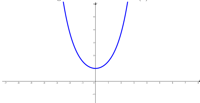
Figura 73: Gráfico de \cosh(x) .
