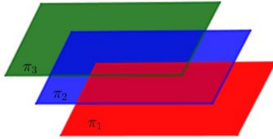
Figura 6: 3 planos paralelos
