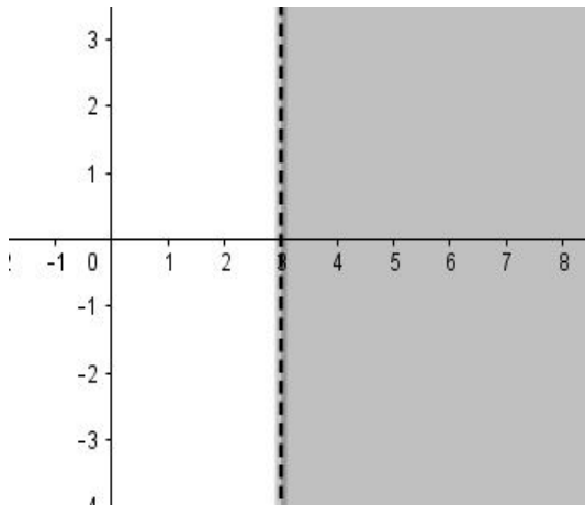
(c) Inequação x > 3
