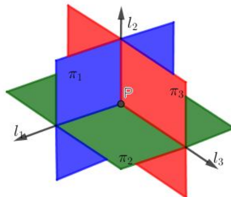
Figura 11: Intersecção em um ponto
