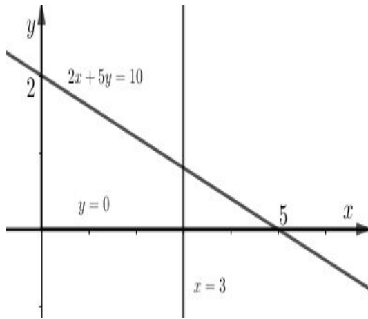
(a) Retas associadas ao sistema
